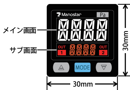
【外観図】
